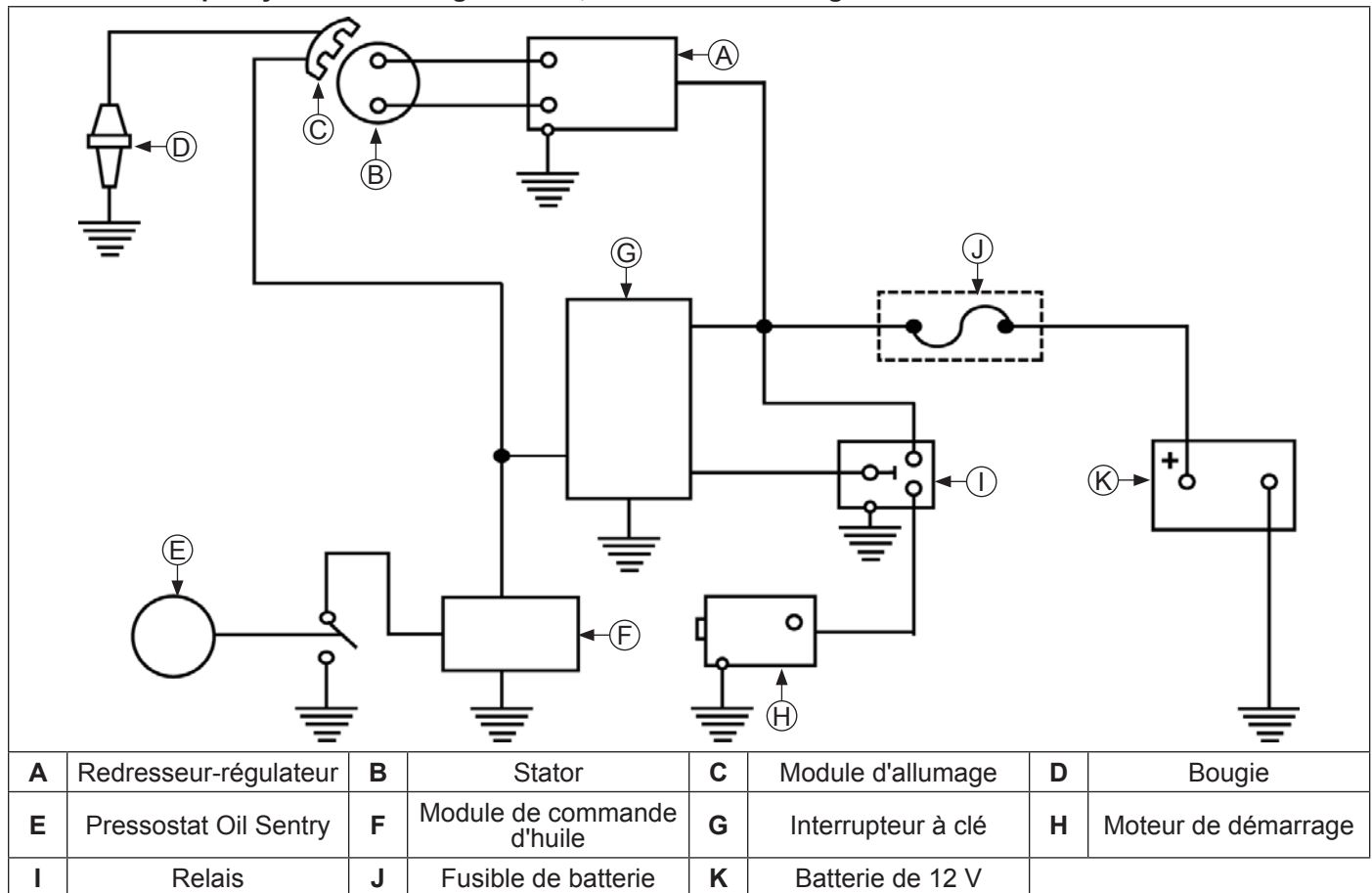
Schéma électrique-système de charge 10/18 A, avec redresseur-régulateur
